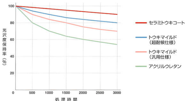
サンシャインウエザオメーター処理
